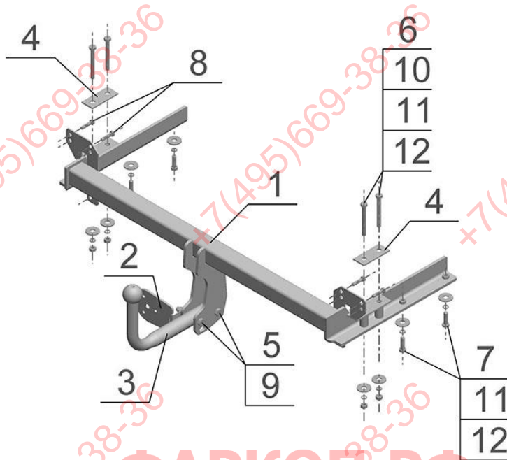
Рис.1. Схема сборки ТСУ.
